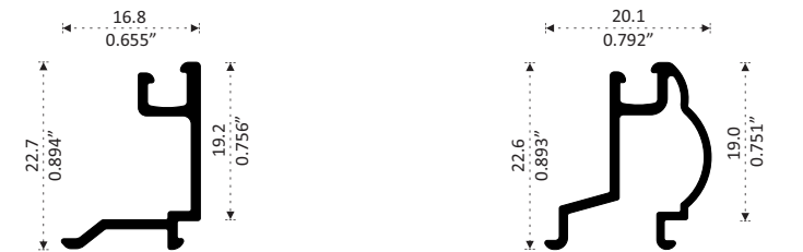
22603 JUNQUILLO CRISTAL DOBLE Longitud 6.10 m
