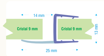
Aleta Lateral Flexible Longitud 2.50 m.
