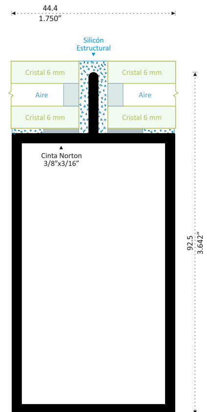
11003 BÁSICO TUBULAR INTEGRAL 3" X 1 3/4" Longitud 6.10 m
