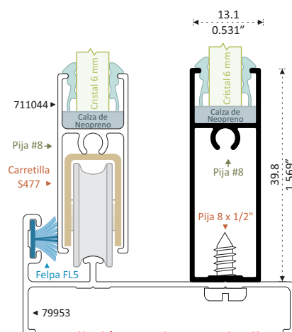
77523 PATENTE ZOCLO FIJO Longitud 6.10 m
