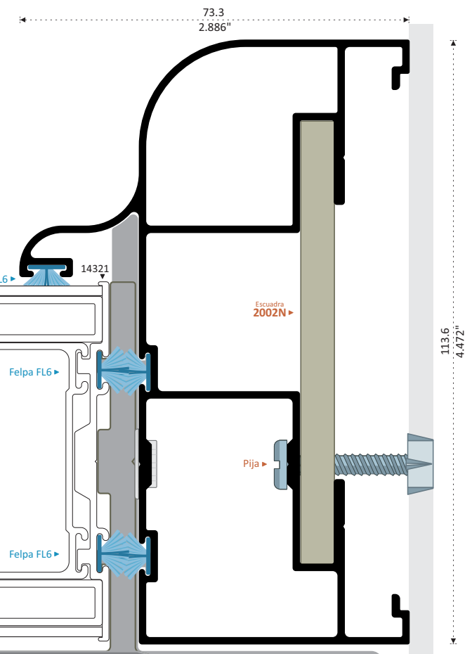
29243 BATIENTE Longitud 6.10 m
