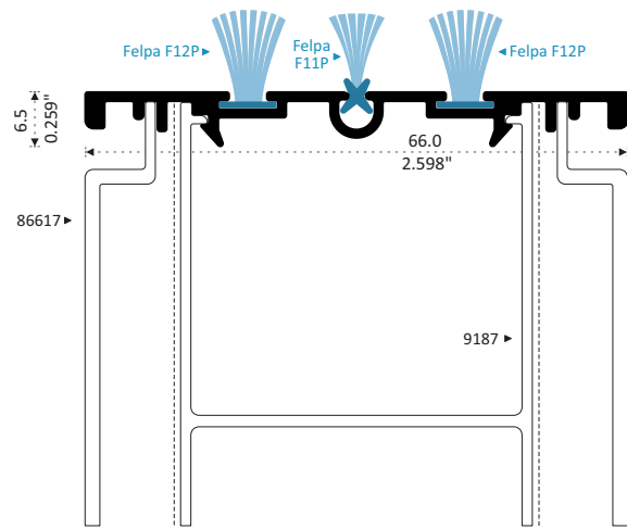
39188 PATENTE SELLO DE HERMETICIDAD SUPERIOR Longitud 3.05 m
