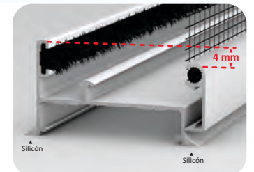
Mosquitero 11763 en Riel
