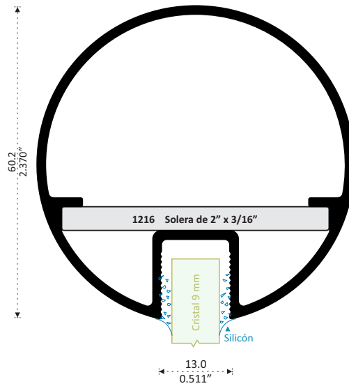
23896 PASAMANOS 2.3" Longitud 6.10 m
