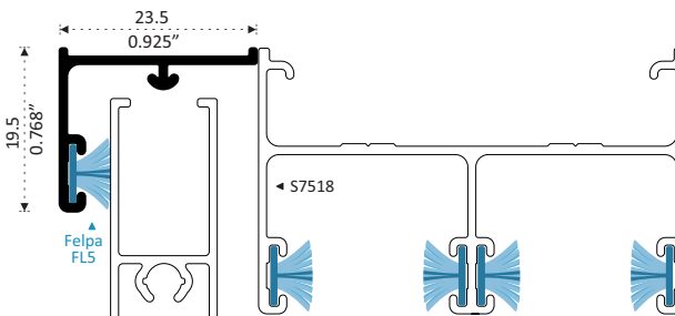
26533 PATENTE MOSQUITERO HORIZONTAL PUERTA Longitud 6.10 m
