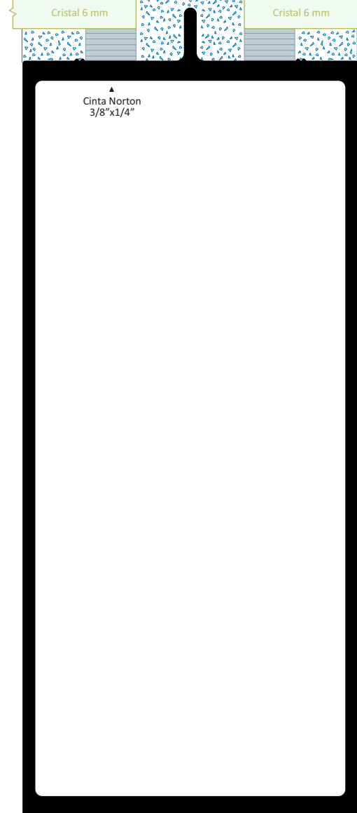
14739 BÁSICO TUBULAR INTEGRAL 6" X 2 1/2" Longitud 6.10 m
