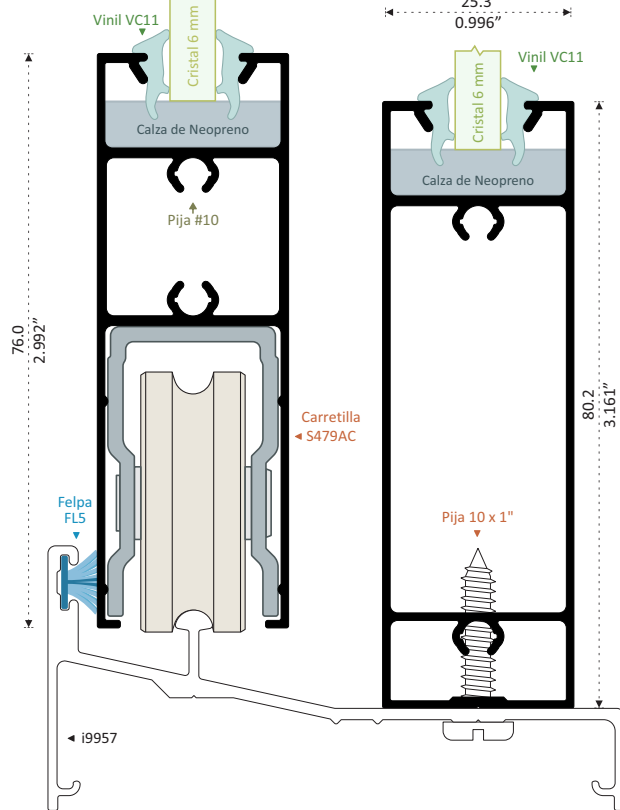
7845 ZOCLO CON BASE Longitud 6.10 m
