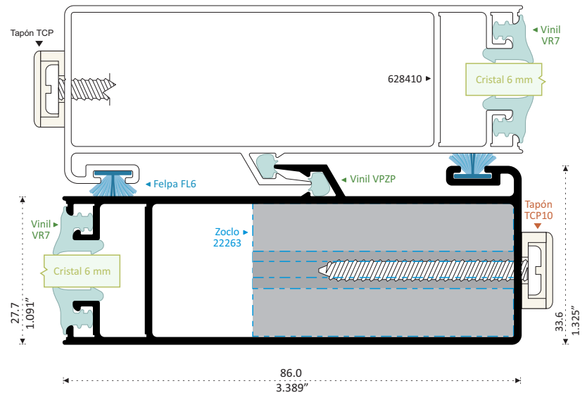
628410 TRASLAPE PUERTA Longitud 5.00 m
