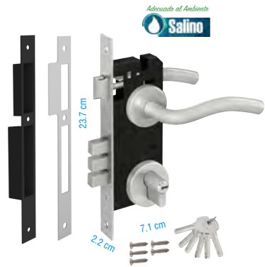
2865P Llave - Llave Cilindro 8 cm
