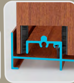
2 Felpas Verticales en Traslapes
