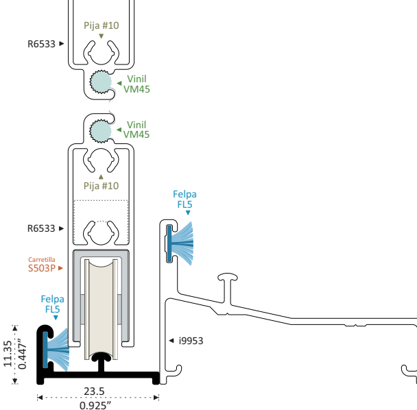
7817 PATENTE RIEL ADAPTADOR MOSQUITERO Longitud 6.10 m
