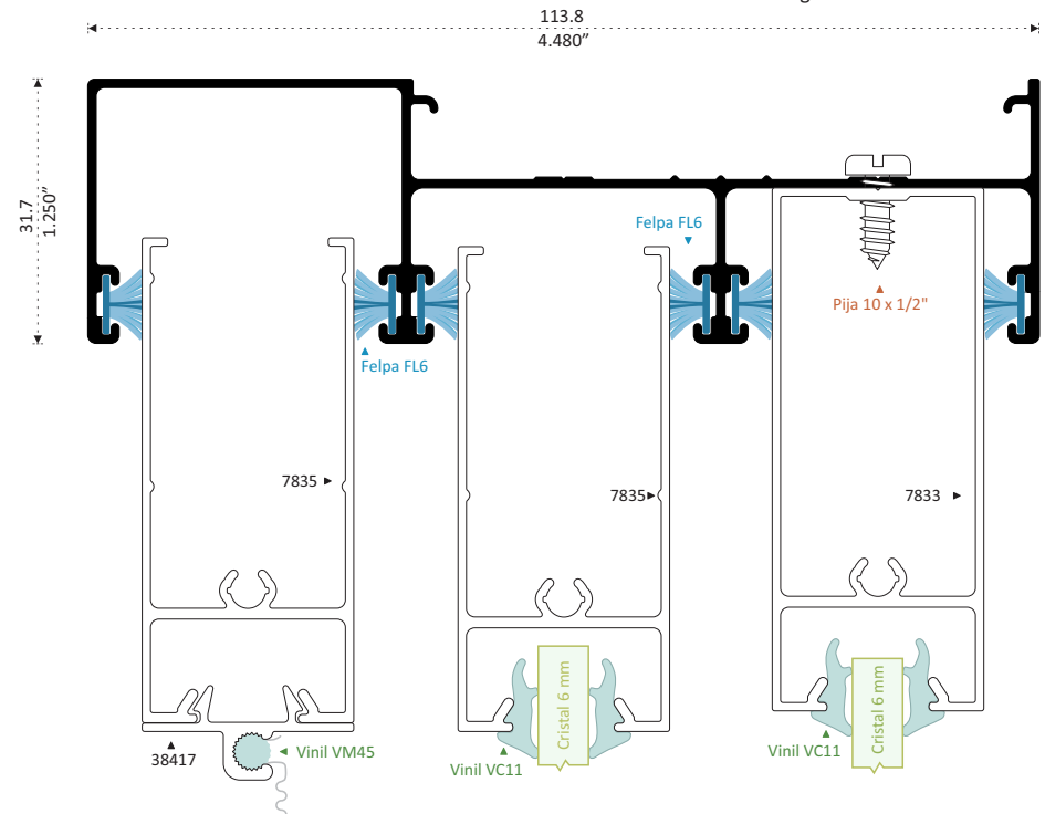
7863 CONTRAMARCO MOSQUITERO CORREDIZO SIN VENAS Longitud 6.10 m
