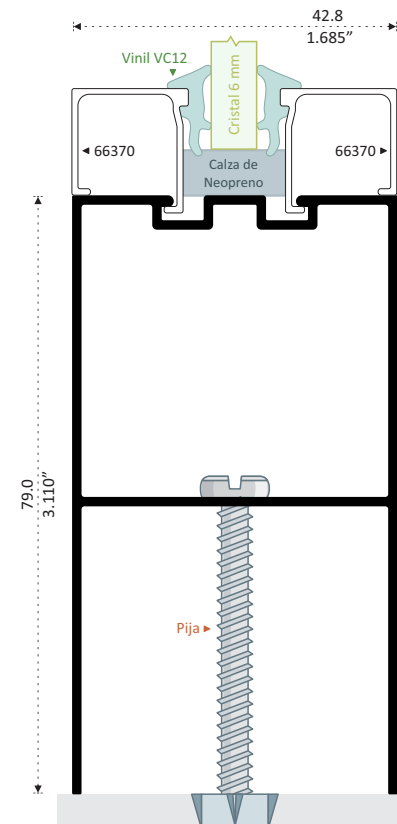
9131 ZOCLO FIJO LIGHT Longitud 6.10 m
