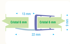
Aleta Lateral Flexible Longitud 2.50 m
