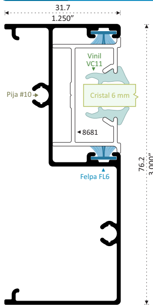
T7826 PATENTE JAMBA Longitud 6.10 m
