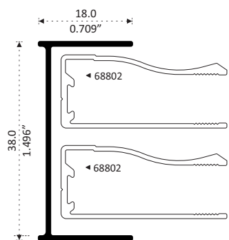
4331 JAMBA Longitud 5.50 m 4331-B 3.77 m 4331-C 3.66 m
