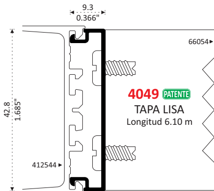
COLOCACIÓN A MURO
