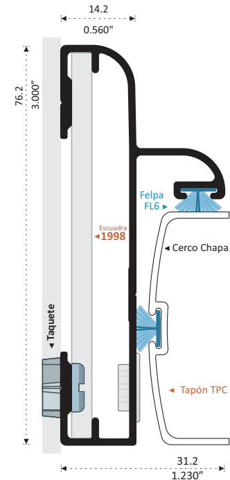
69244 BATIENTE COLONIAL Longitud 6.10 m
