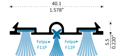
19188 SELLO DE HERMETICIDAD 3 FELPAS Longitud 6.10 m 19188-C 3.05 m SHT 1.00 m
