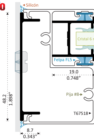
64052 MOLDURA DE FIJACIÓN Longitud 6.10 m TF2 10 cm
