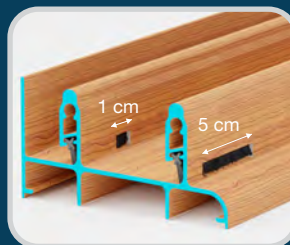
Aumentan la Hermeticidad: - Aislamiento Acústico - Resistencia a Viento - Filtra Polvo - Salida de Agua - Impide Entrada de Insectos Riel Inferior Incluye Drenes cada 40 cm Colocar Felpa F11P
