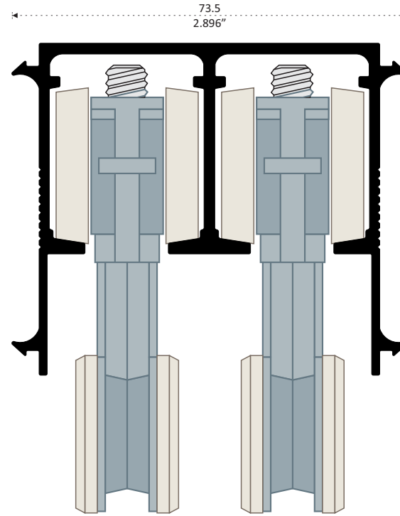
10020 PATENTE RIEL SUPERIOR Longitud 6.10 m
