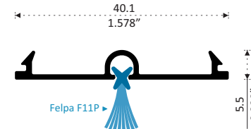
49188 SELLO DE HERMETICIDAD 1 FELPA Longitud 6.10 m TH 1.00 m
