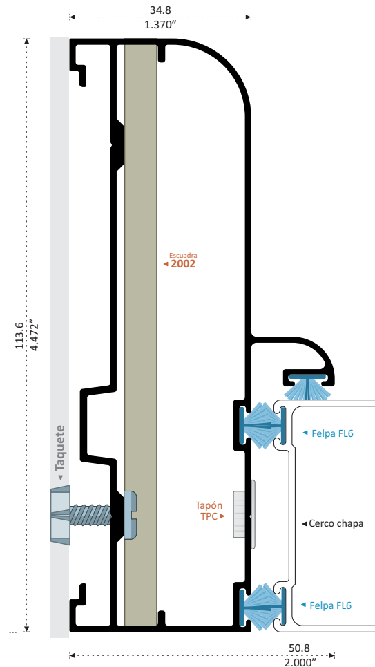
9242 BATIENTE COLONIAL Longitud 6.10 m
