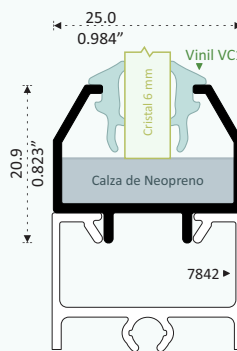
614702 ADAPTADOR BISELADO Longitud 6.10 m
