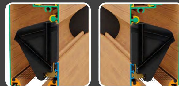
Sello Hermético por sus 2 Tapas Laterales de 3 Felpas con Aletas
