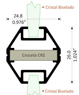
8267 PATENTE INTERMEDIO BISELADO Longitud 6.10 m
