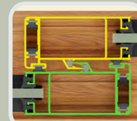
Hermeticidad entre Traslapes por 2 Vinilos VPZP y 6 Felpas
