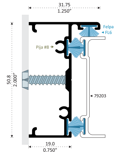
55844 BATIENTE 2" Longitud 6.10 m
