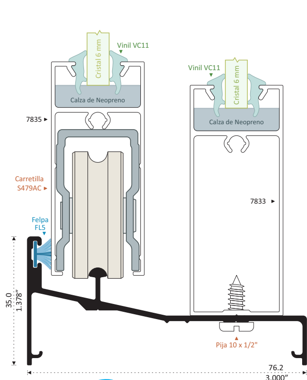
NUEVO i9957 RIEL 3" CON INCLINACIÓN Longitud 6.10 m
