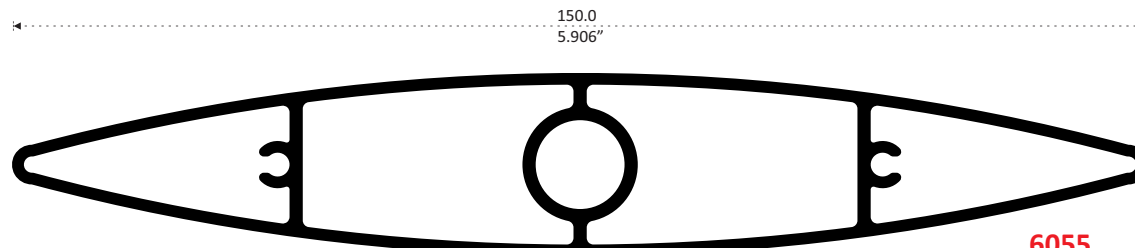
6055 ROMPE VISTA Longitud: 6.10 m
