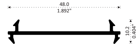
7793 MOLDURA UNIÓN Longitud 6.10 m
