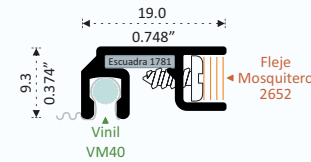
11096 MOSQUITERO DESMONTABLE Longitud 6.10 m
