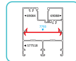
7793 MOLDURA UNIÓN Longitud 6.10 m
