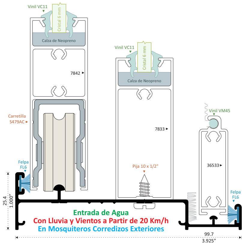
9272 PATENTE RIEL CON MOSQUITERO EXTERIOR Longitud 6.10 m
