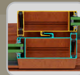
Perfiles Reforzados de 5 Pulgadas
