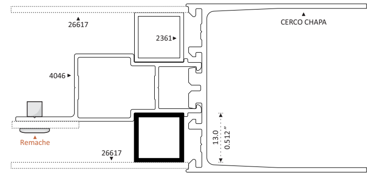
2361 CUADRADO 13 mm Longitud 6.10 m
