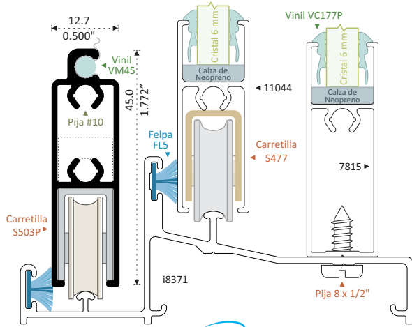
R6533 MOSQUITERO HORIZONTAL DOBLE VENA Longitud 6.10 m
