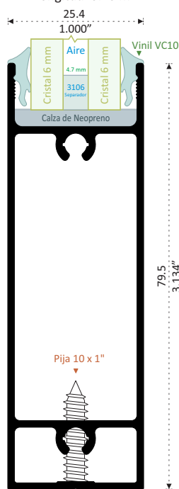
9962 NUEVO ZOCLO FIJO Longitud 6.10 m
