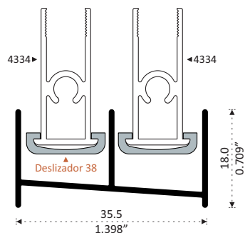
4332 GUÍA INFERIOR Longitud 6.10 m
