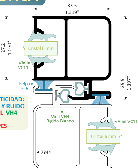
NUEVO 7844 PATENTE TRASLAPE Longitud 6.10 m
