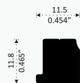
34717 BARRA SOPORTE 1 Longitud 6.10 m Drenes de 1 cm cada 40 cm
