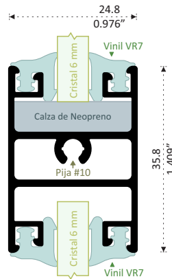
13842 PATENTE INTERMEDIO Longitud 6.10 m
