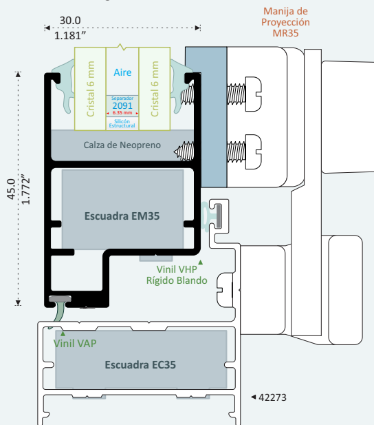
22277 PATENTE MARCO CRISTAL DOBLE Longitud 6.10 m
