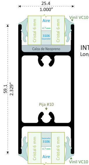
9962 NUEVO ZOCLO FIJO Longitud 6.10 m
