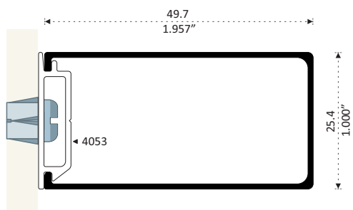
72521 ROMPE VISTA Longitud 6.10 m
