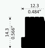
34719 BARRA SOPORTE 3 Longitud 6.10 m Drenes de 5 cm cada 40 cm
