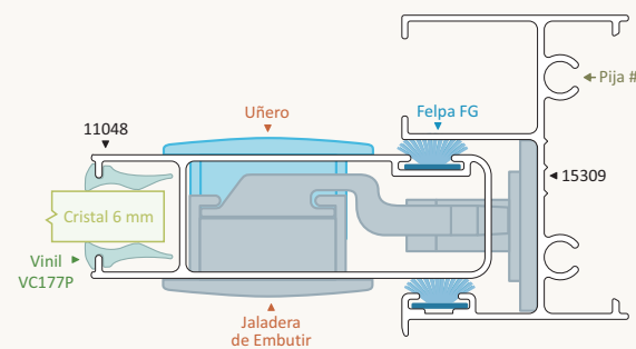
11048 PATENTE CERCO Y TRASLAPE PUERTA Longitud 6.10 m
