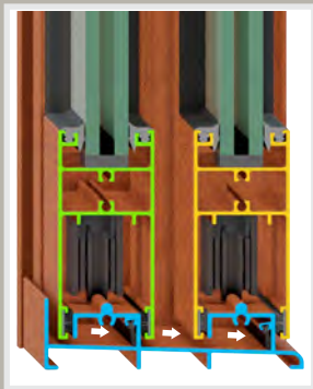
Mejor Salida de Agua por: - Riel con Pared Interior Alta - Inclinación de Riel - Drenes Inferiores
