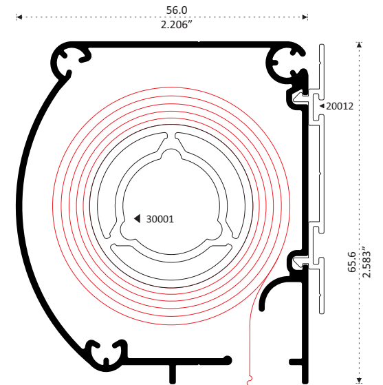
20011 PATENTE CAJÓN PUERTA Longitud 6.10 m 20011-C 3.05 m
