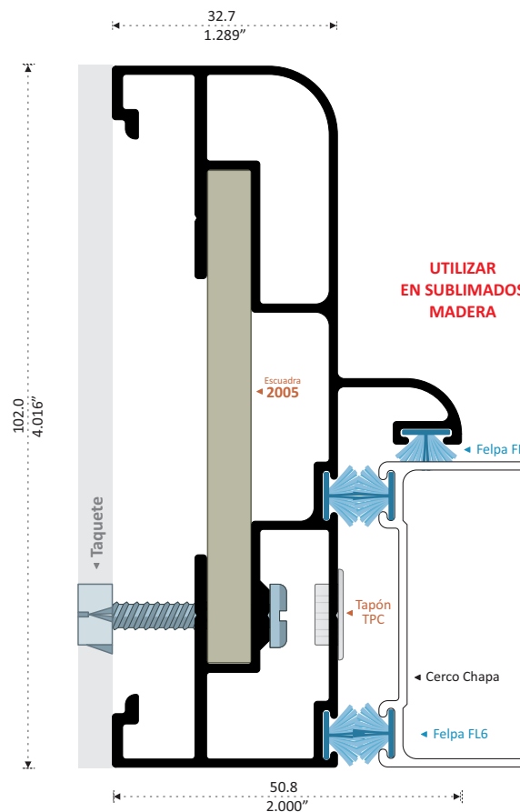
22619 PATENTE BATIENTE COLONIAL Longitud 6.10 m
