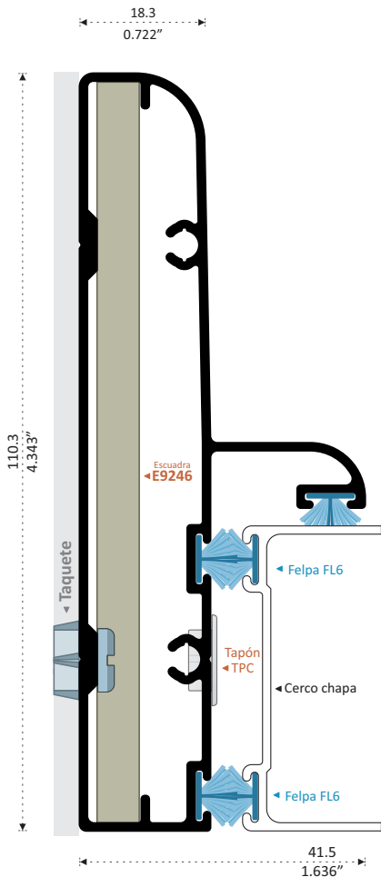
9246 PATENTE BATIENTE COLONIAL Longitud 6.10 m
