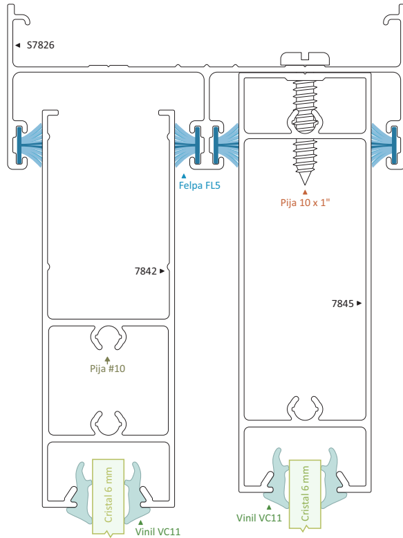
7842 ZOCLO PUERTA Longitud 6.10 m
