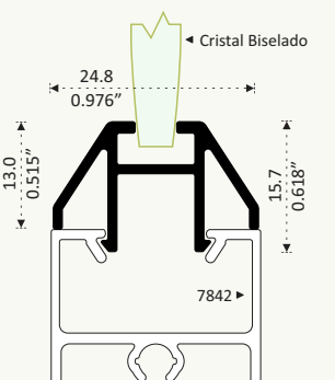
8265 PATENTE ADAPTADOR BISELADO Longitud 6.10 m
