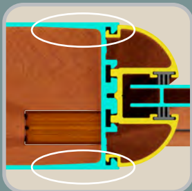
Cerco Chapa con Refuerzos en Paredes Interiores Dando Resistencia al Apretar el Tensor
