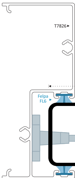
17847 CERCO CHAPA GRAN VISTA Longitud 6.10 m 17847-C 4.60 m
