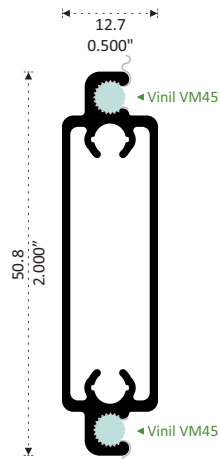
7101 INTERMEDIO MOSQUITERO Longitud 6.10 m
