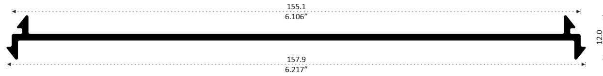
23618 MOLDURA UNIÓN Longitud: 6.10 m
