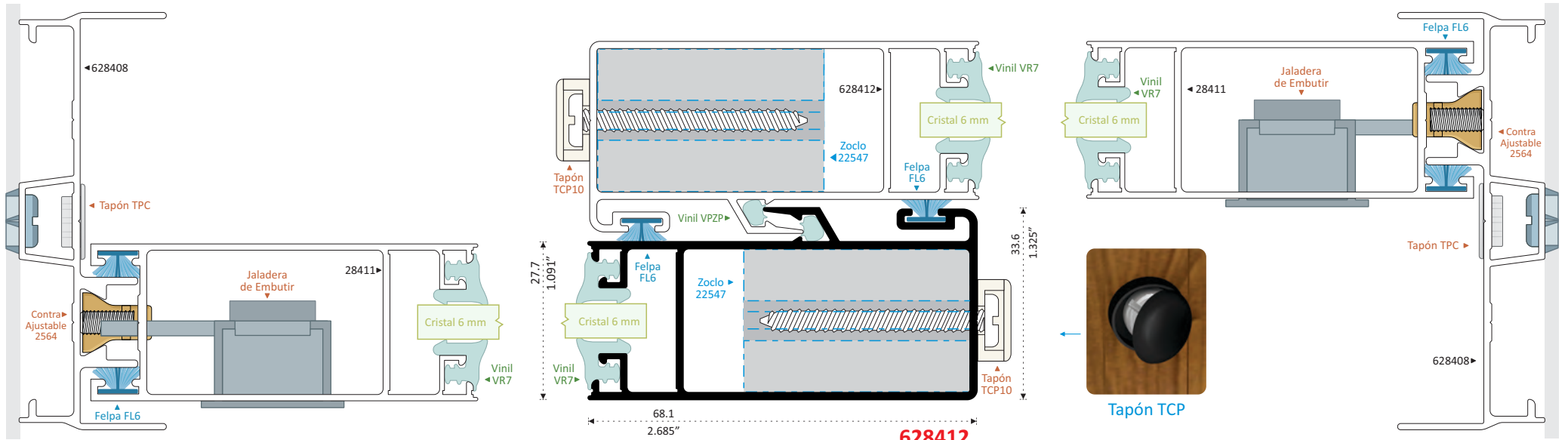
628412 TRASLAPE VENTANA Longitud 6.10 m
