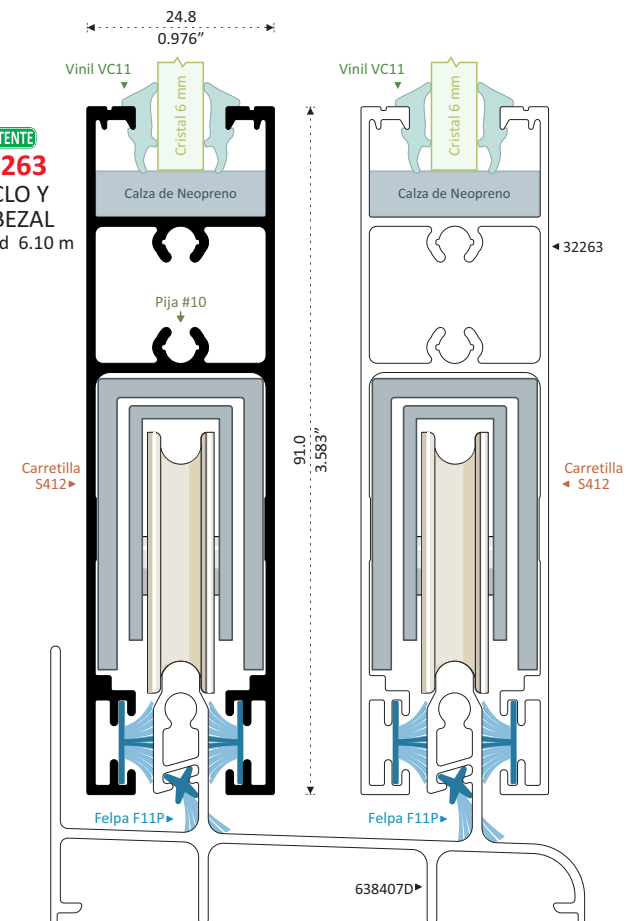
Ensambla con Línea Fija
