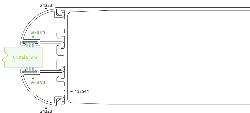
5117 BATIENTE DESLIZABLE Longitud 6.10 m
