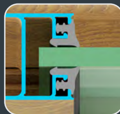
Doble Vinil Respaldo Aumenta Aislamiento Acústico
