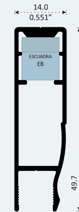
Marco Armado con Escuadra Tradicional 1573
