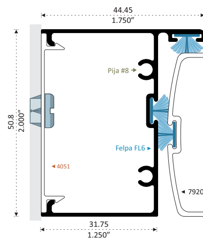
78591 PATENTE BATIENTE 2" Longitud 6.10 m
