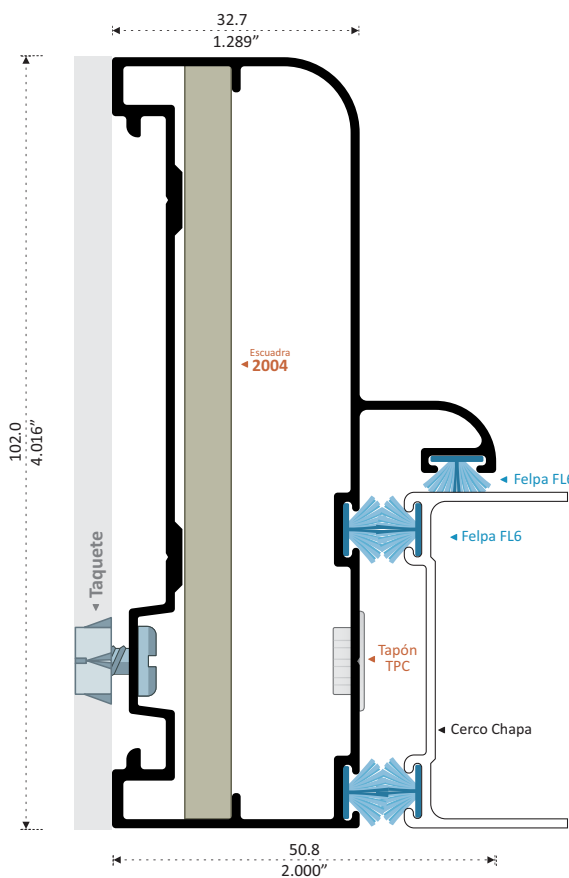
12619 PATENTE BATIENTE COLONIAL Longitud 6.10 m
