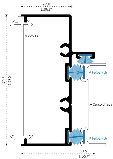
12757 BATIENTE Longitud 6.10 m
