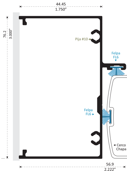
9116 BATIENTE Longitud 6.10 m
