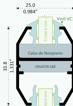
614918 INTERMEDIO BISELADO Longitud 6.10 m
