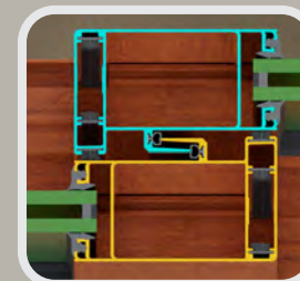
Hermeticidad entre Traslapes por 2 Vinilos Hongo y 6 Felpas
