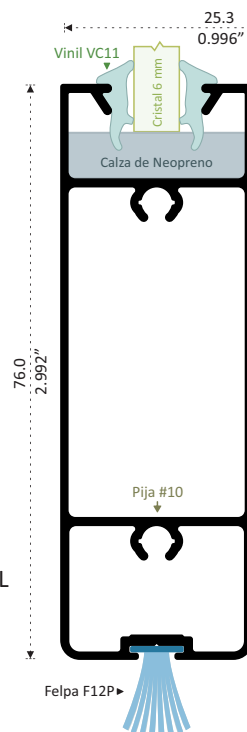
7839 PATENTE ZOCLO CABEZAL Longitud 6.10 m 7839-C 3.05 m ZEC 1.00 m
