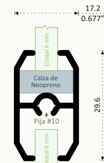
12394 BARROTILLO Longitud 6.10 m
