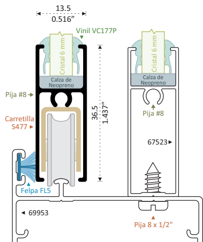
611044 ZOCLO Y CABEZAL Longitud 6.10 m
