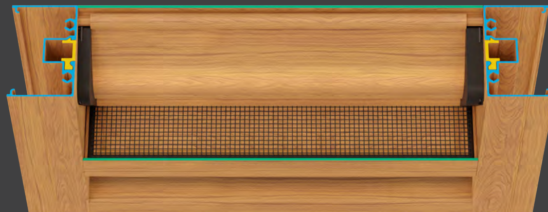
Sello Hermético por sus 2 Tapas Laterales de 3 Felpas con Aletas
