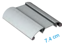
REGLA DE CORTE Cortado del Perfil 5019 1108 1.92 m. 1107 2.90 m.
