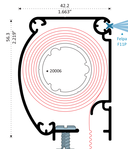
20010 PATENTE CAJÓN MOSQUITERO Longitud 6.10 m 20010-C 3.05 m
