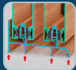
Resistencia de 4 Puntos de Apoyo para Cristales Pesados
