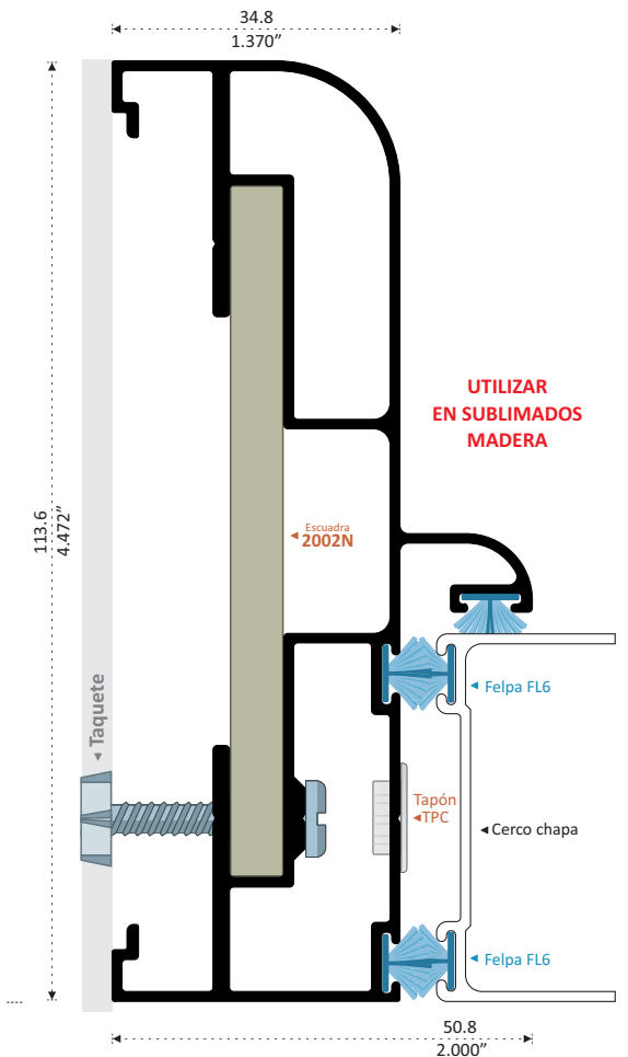
19242 BATIENTE COLONIAL Longitud 6.10 m
