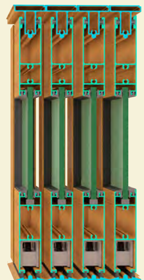
Riel Sencillo a Piso
