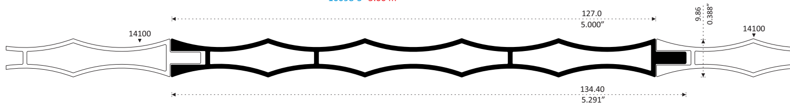
14100 PATENTE DUELA CINCO ONDAS DOBLE VISTA 5" Longitud : 6.10 m 14100-5 5.00 m
