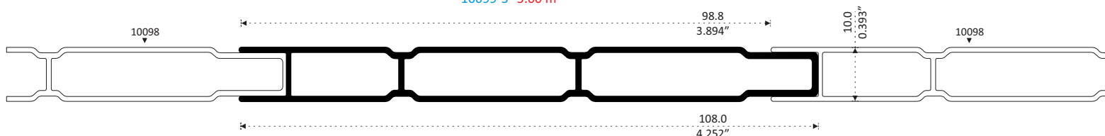
10098 PATENTE DUELA DOBLE VISTA Longitud 6.10 m 10098-5 5.00 m
