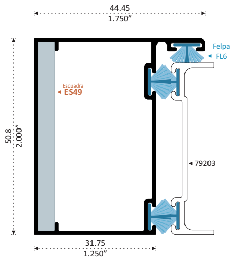
28591 BATIENTE Longitud 6.10 m
