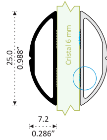
8272 MARQUETERÍA EXPUESTA CURVA Longitud 6.10 m
