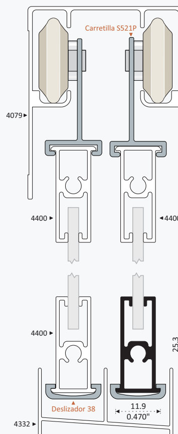
4400 MARCO HORIZONTAL Longitud 6.10 m 4400-C 3.05 m
