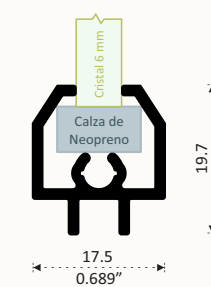
12395 RESERCADO Longitud 6.10 m
