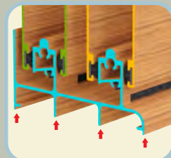
Resistencia de con 4 Puntos de Apoyo para Cristales Pesados
