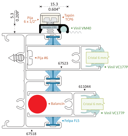
11763 MOSQUITERO FIJO Longitud 6.10 m
