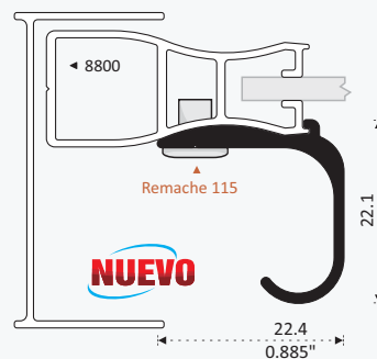
4200 JALADERA TROMPA DE ELEFANTE Longitud 3.05 m JT42 10 cm
