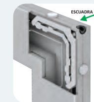
Marco Armado con Escuadra de Botón EB AJUSTA Y CIERRA EL CORTE
