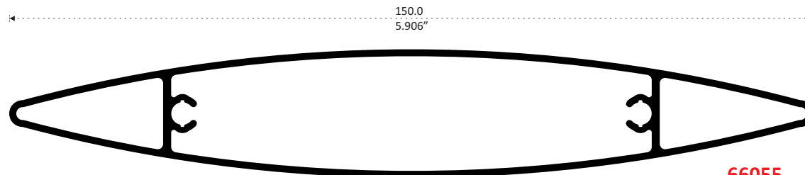
66055 ROMPE VISTA Longitud: 6.10 m
