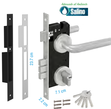
2868P Llave - Llave Cilindro 8 cm
