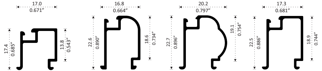
412543 PATENTE JUNQUILLO Longitud 6.10 m
