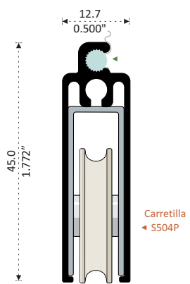
6533 PATENTE MOSQUITERO HORIZONTAL VENTANA Longitud 6.10 m
