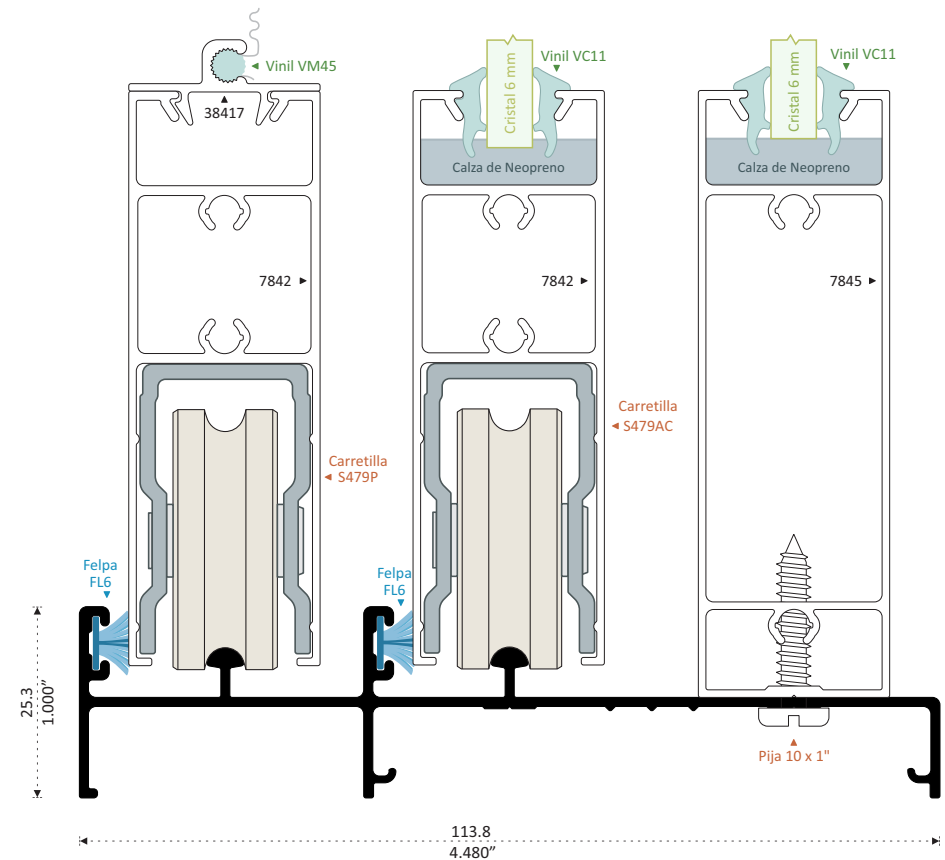
9275 RIEL CON MOSQUITERO INTERIOR Longitud 6.10 m
