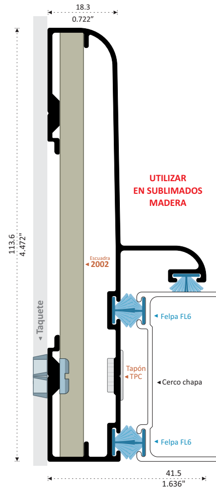
69246 BATIENTE COLONIAL Longitud 6.10 m
