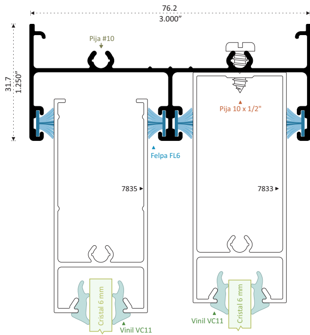
7826 CONTRAMARCO Longitud 6.10 m 7826-C 4.60 m
