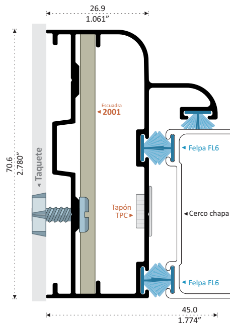
12618 BATIENTE COLONIAL Longitud 6.10 m
