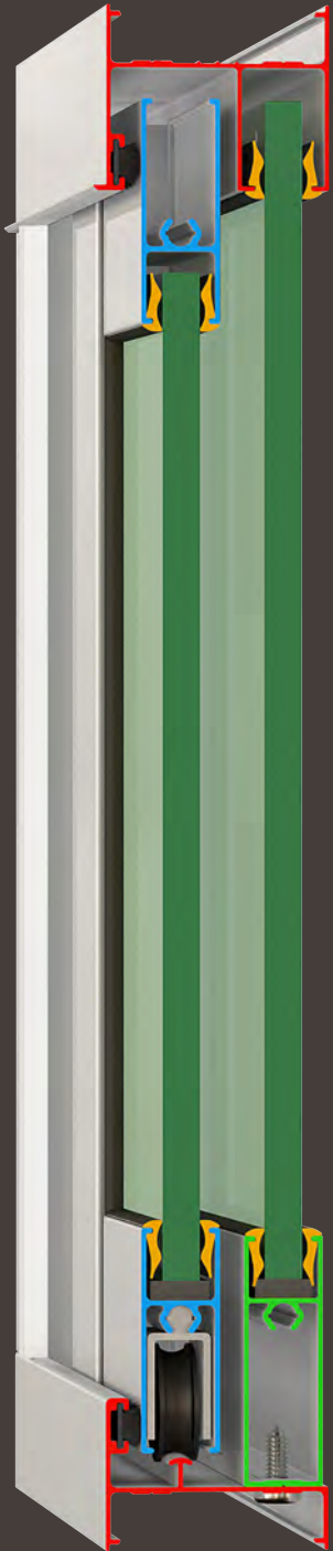
Pijas sin Contacto con el Cristal
