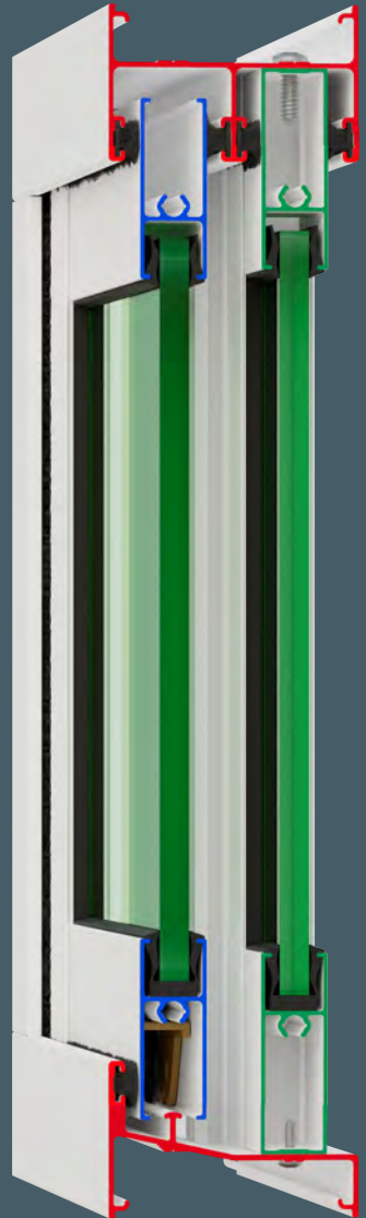
Armado Horizontal Superior
