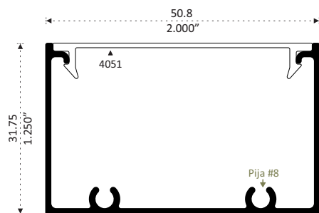
68591 CANAL Longitud 6.10 m
