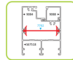
7792 MOLDURA UNIÓN Longitud 6.10 m
