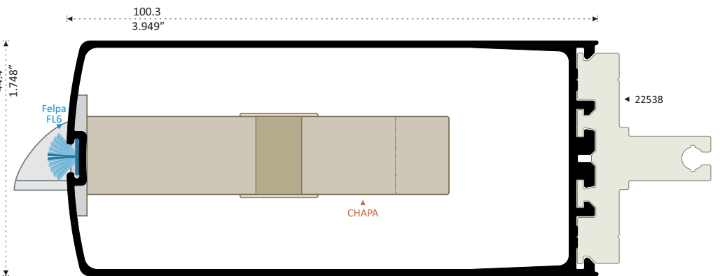
46901 PATENTE CERCO CHAPA Longitud: 5.00 m
