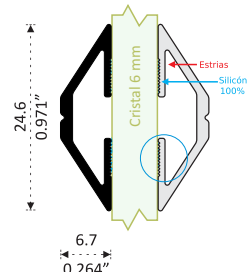
8264 MARQUETERÍA EXPUESTA BISELADA Longitud 6.10 m
