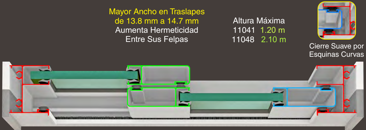
Zoclo de Hoja Fija con Mayor Resistencia ante Ráfagas de Viento
