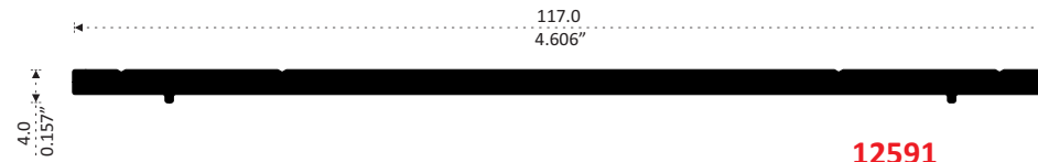
12591 TAPA BISAGRA Longitud 6.10 m Clave 3125 33 cm
