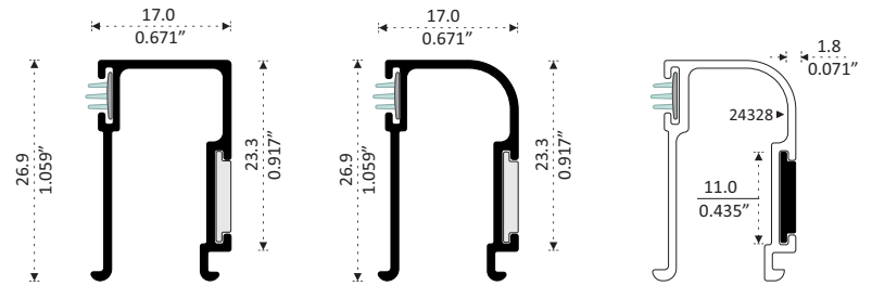
24327 PATENTE JUNQUILLO MARQUETERÍA Longitud 6.10 m
