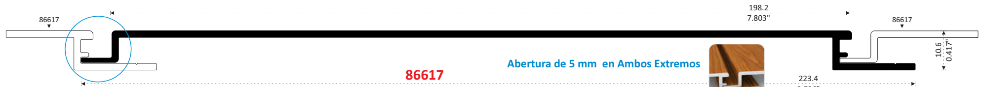
96617 PATENTE DUELA LISA Longitud: 6.10 m
