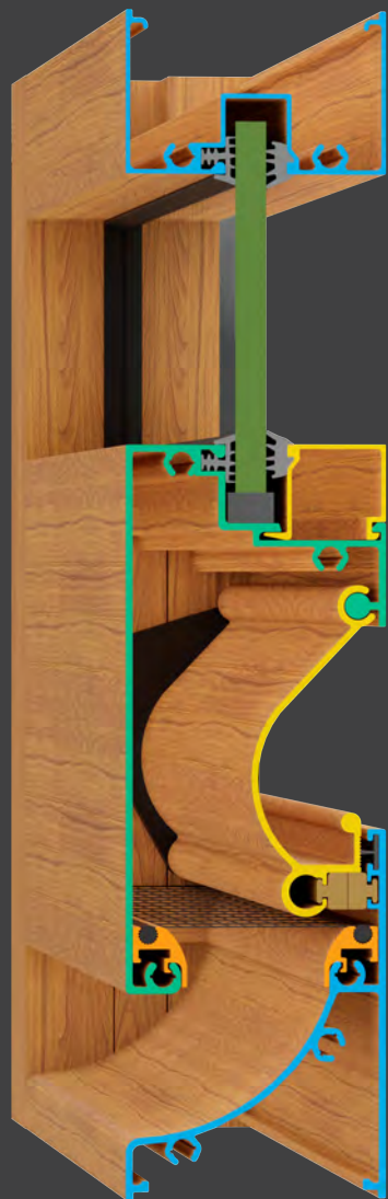
Mosquitero Horizontal Oculto
