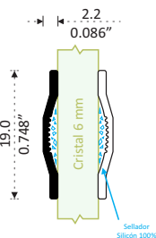
81642 CUADRÍCULA EXPUESTA Longitud 6.10 m
