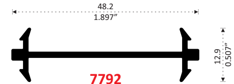
7792 MOLDURA UNIÓN Longitud 6.10 m
