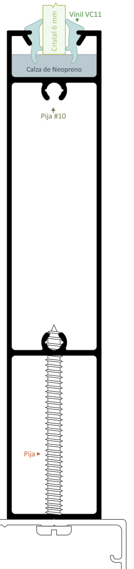
17840 ZOCLO FIJO 5" Longitud 6.10 m
