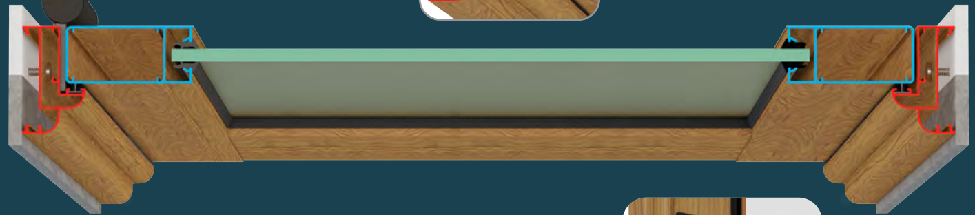
Batiente y Cerco Chapa con Entradas para Barra Refuerzo
