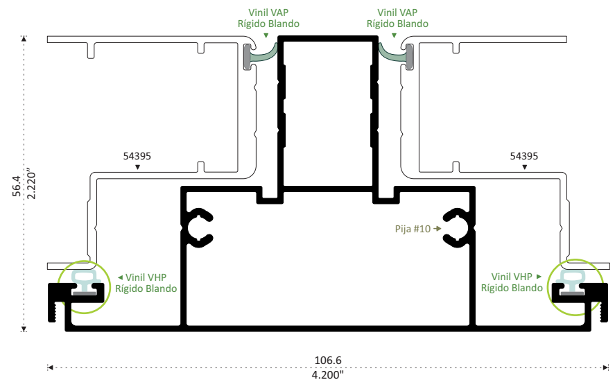
34397 INTERMEDIO Longitud 6.10 m
