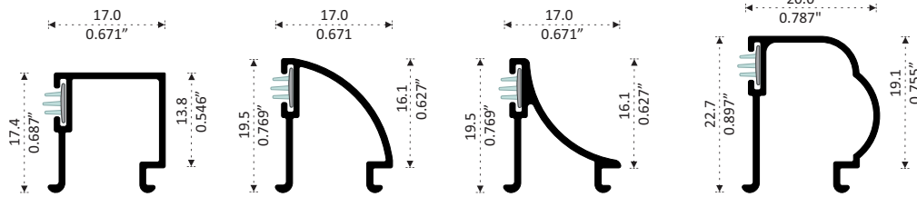
76370 JUNQUILLO Longitud 6.10 m
