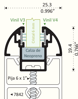
8269 ADAPTADOR CURVO Longitud 6.10 m
