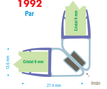
Burbuja Flexible con Imán Longitud 2.50 m.
