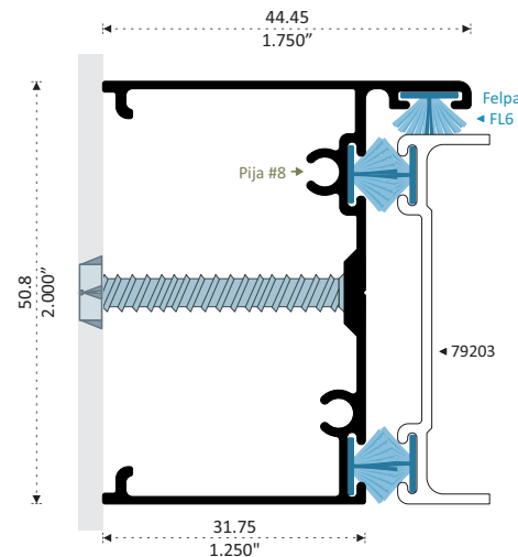
58591 BATIENTE 2" Longitud 6.10 m
