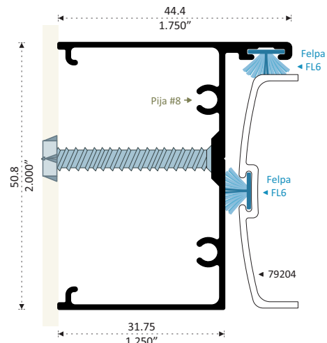
48591 BATIENTE 2" Longitud 6.10 m
