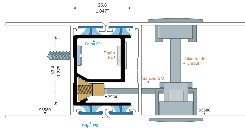
13637 PATENTE ADAPTADOR Longitud 6.10 m
