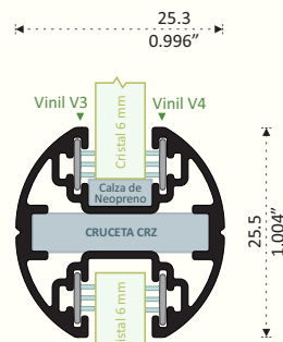
8271 PATENTE INTERMEDIO CURVO Longitud 6.10 m
