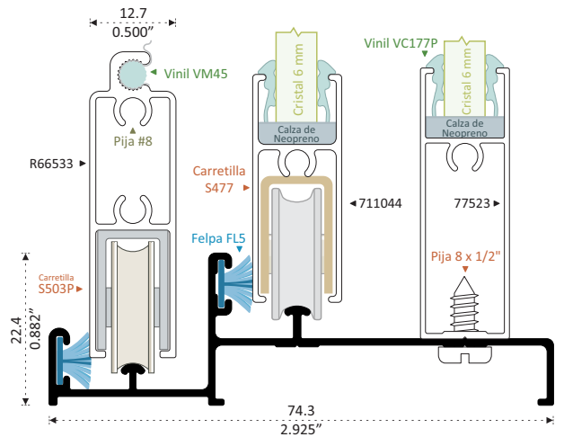
78371 RIEL MOSQUITERO INTERIOR Longitud 6.10 m
