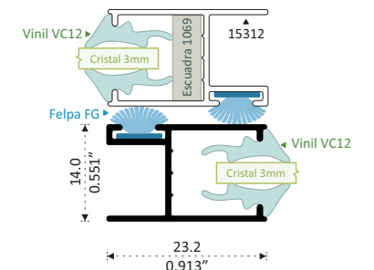
15312 CERCO Y TRASLAPE VENTANA Longitud 6.10 m
