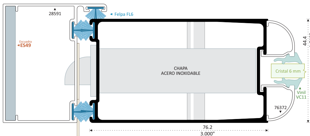
79205 CERCO CHAPA 3" Longitud 4.60 m 79205-L 6.10 m
