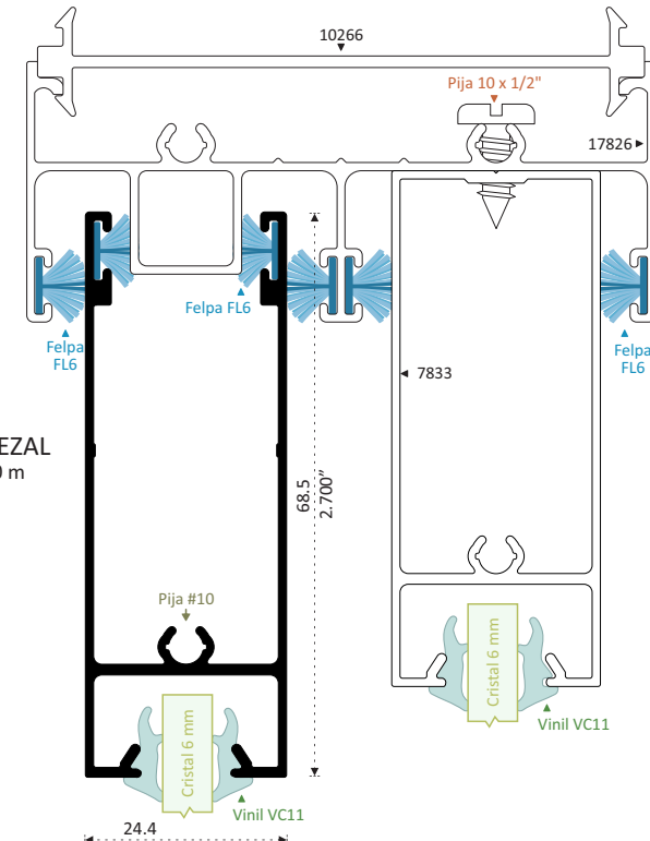
27842 ZOCLO FIJO Longitud 6.10 m
