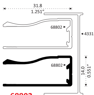
68802 MARCO Longitud 6.10 m 68802-C 3.66 m
