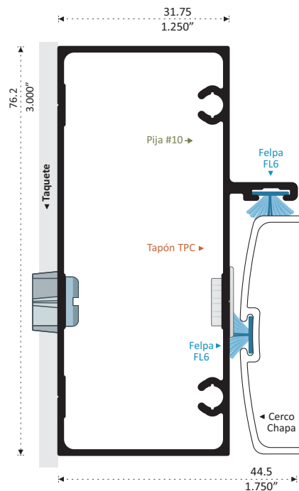
9133 BATIENTE Longitud 6.10 m
