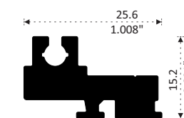
12538 BARRA DE ARMADO Longitud 3.03 m
