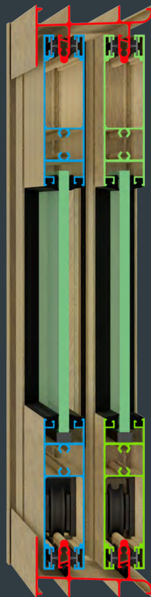
Mejor Salida de Agua por: - Riel con Pared Interior Alta - Inclinación de Riel - Drenes Inferiores
