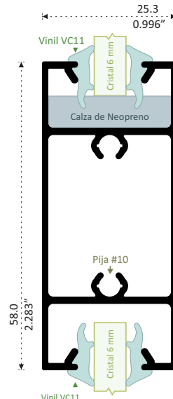
7837 PATENTE INTERMEDIO Longitud 6.10 m 7837-C 3.05 m IPF 0.87 m
