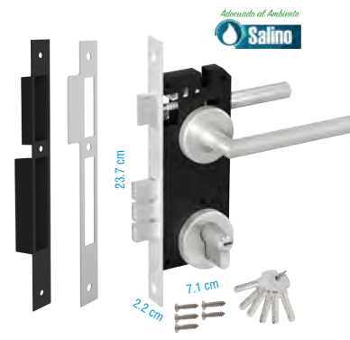
2822P Llave - Llave Cilindro 8 cm
