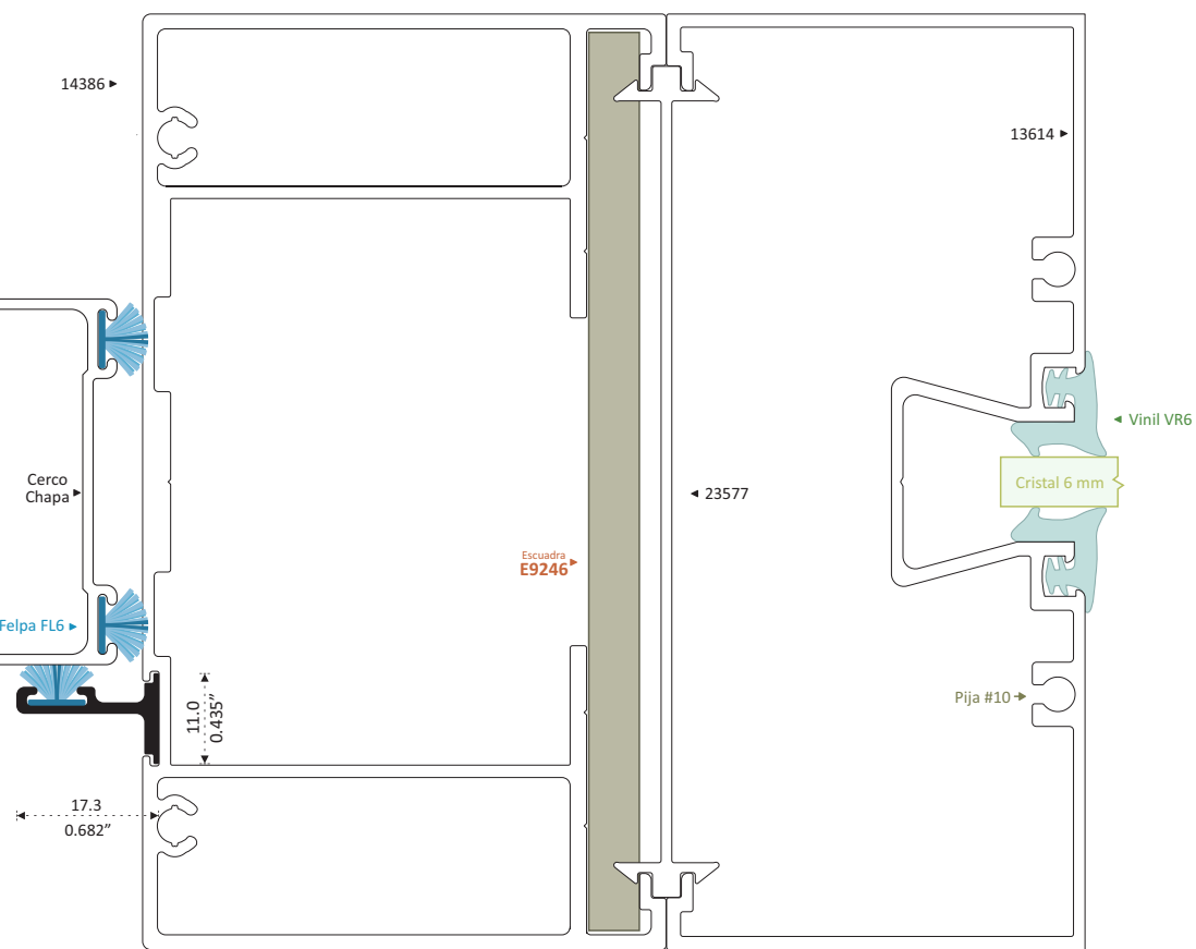
5117 BATIENTE DESLIZABLE Longitud 6.10 m
