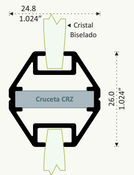
8267 PATENTE INTERMEDIO BISELADO Longitud 6.10 m
