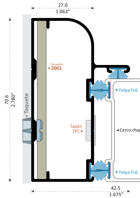
22757 BATIENTE COLONIAL Longitud 6.10 m
