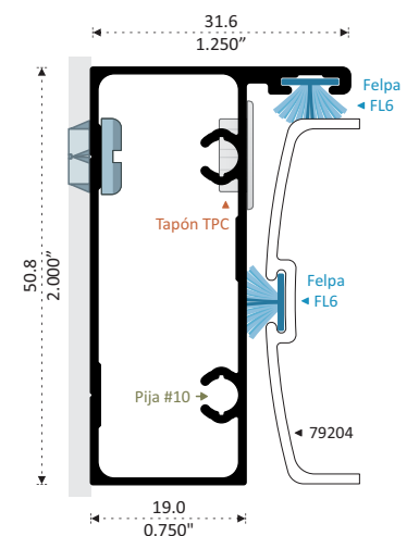
45844 BATIENTE Longitud 6.10 m
