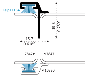
10220 ADAPTADOR Longitud 6.10 m
