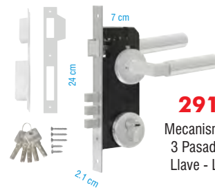
2866 Mecanismo de 3 Pasadores Llave - Llave
