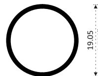
2108 REDONDO DE 3/4" Longitud 6.10 m
