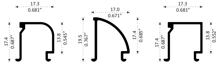
32576 JUNQUILLO COLONIAL Longitud 6.10 m
