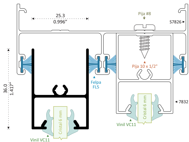
7836 CABEZAL Longitud 6.10 m
