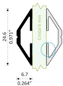
8264 MARQUETERÍA EXPUESTA BISELADA Longitud 6.10 m
