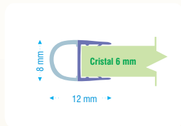
Burbuja Flexible Longitud 2.50 m
