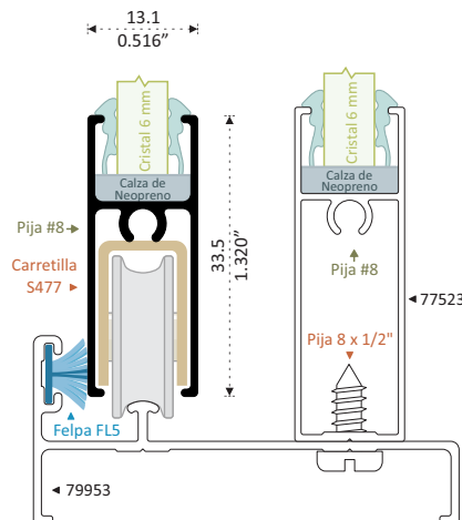
711044 ZOCLO Y CABEZAL Longitud 6.10 m
