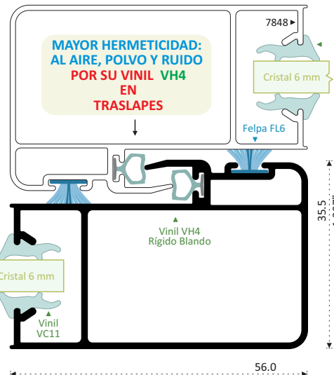
NUEVO 7848 PATENTE TRASLAPE Longitud 4.60 m 7848-5.1 5.10 m 7848-L 6.10 m
