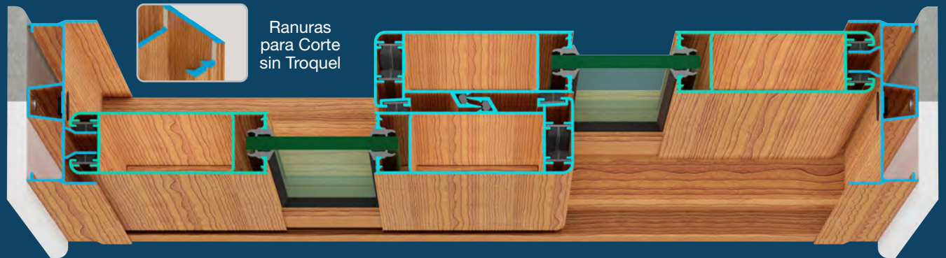
2 Felpas Horizontales en Zoclo
