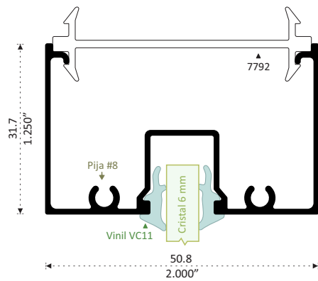
69083 BOLSA Longitud 6.10 m
