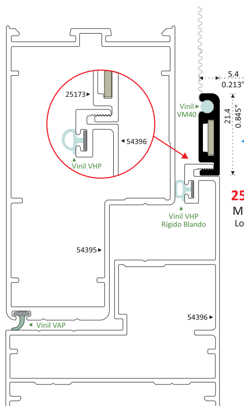
Estrías en Perfil y Vinil Logrando Mayor Tensión a la Tela Mosquitero Sin Salirse de su Lugar
