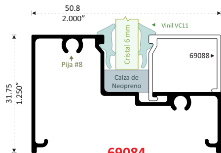
69084 ESCALONADO Longitud 6.10 m
