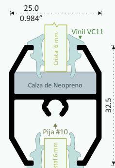
14918 INTERMEDIO BISELADO Longitud 6.10 m
