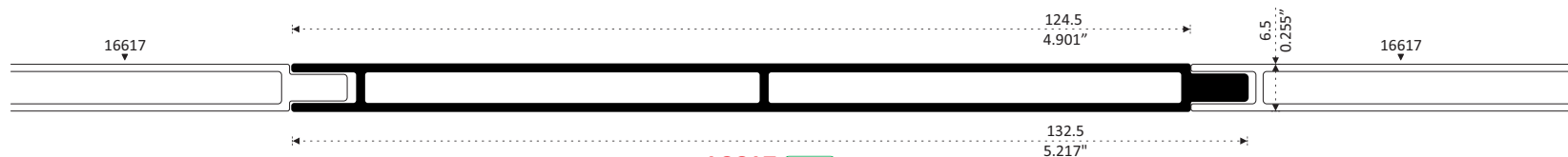
16617 PATENTE DUELA LISA DOBLE VISTA 5" Longitud : 6.10 m 16617-C 4.60 m 16617-5 5.00 m
