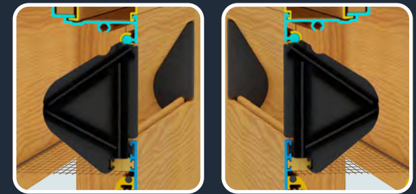
Sello Hermético por sus 2 Tapas Laterales de 3 Felpas con Aletas
