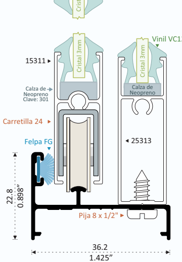
15310 RIEL Longitud 6.10 m
