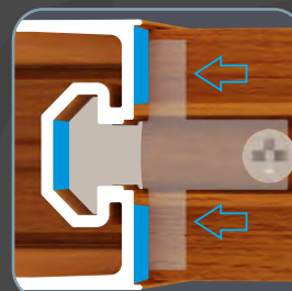
Paredes de Esfuerzo a la Compresión
