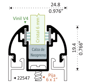
8268 PATENTE ADAPTADOR CURVO Longitud 6.10 m
