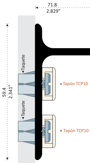
11560 PATENTE SOPORTE PASAMANOS Longitud 6.10 m
