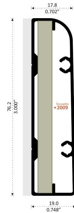
9245 PATENTE MARCO COLONIAL Longitud 6.10 m
