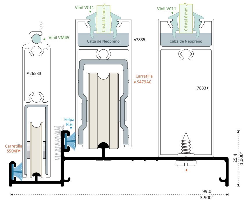
9274 PATENTE RIEL CON MOSQUITERO INTERIOR Longitud 6.10 m
