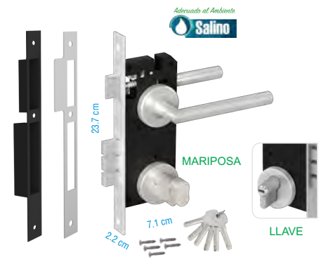
2822M Llave - Mariposa Cilindro 8 cm
