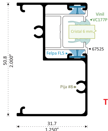
64052 MOLDURA DE FIJACIÓN Longitud 6.10 m TF2 10 cm
