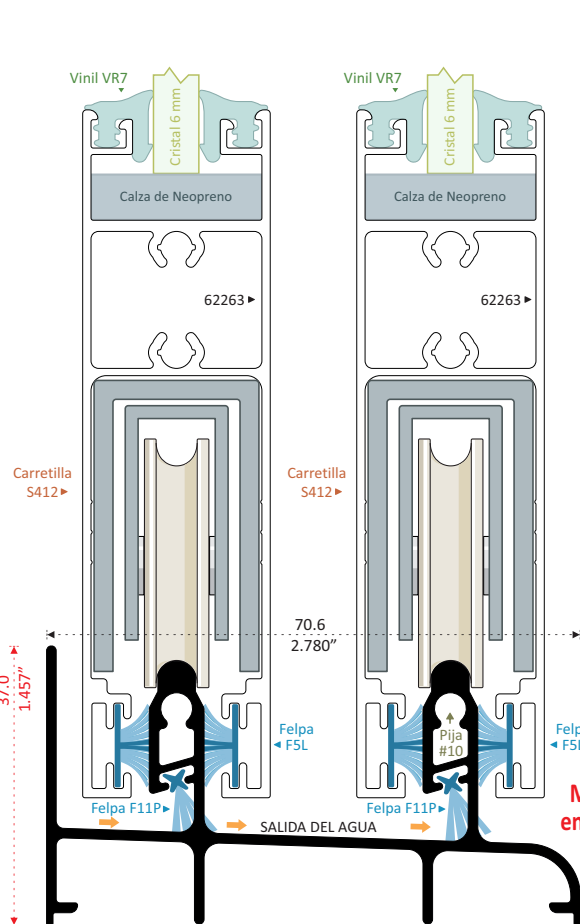
62263 PATENTE ZOCLO Y CABEZAL Longitud 6.10 m
