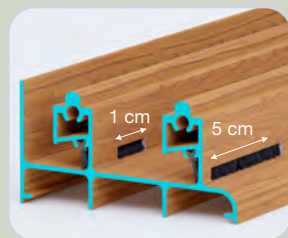
Aumentan la Hermeticidad: - Aislamiento Acústico - Resistencia a Viento - Filtra Polvo - Salida de Agua - Impide Entrada de Insectos
