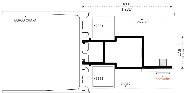
4046 SOPORTE Longitud: 6.10 m
