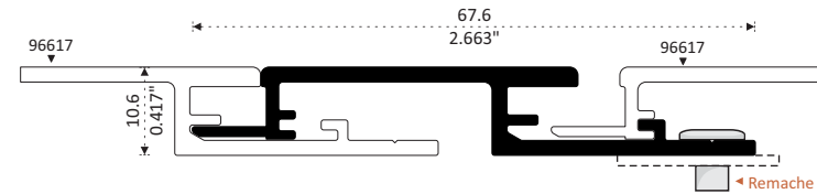
8519 DUELA Longitud: 6.10 m
