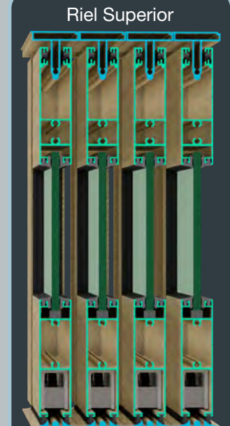
Riel Sencillo a Piso
