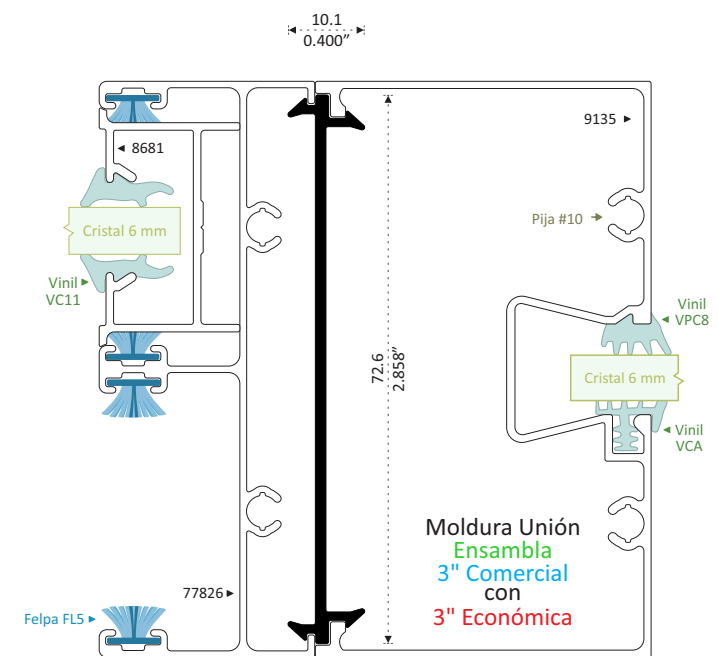
10265 MOLDURA UNIÓN Longitud 6.10 m
