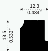
34718 BARRA SOPORTE 2 Longitud 6.10 m Drenes de 5 cm cada 40 cm
