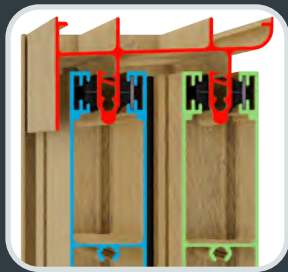
Riel Doble Guía Opcional Dos Hojas Móviles
