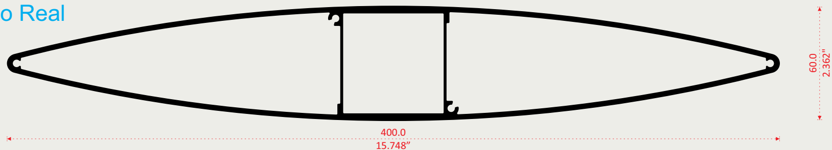
6082 ROMPE VISTA Longitud : 6.10 m.
