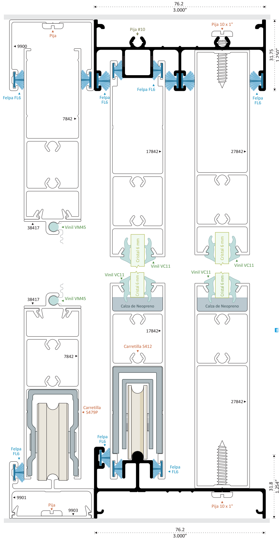
NUEVO 19957 PATENTE RIEL HERMÉTICO Longitud 6.10 m
