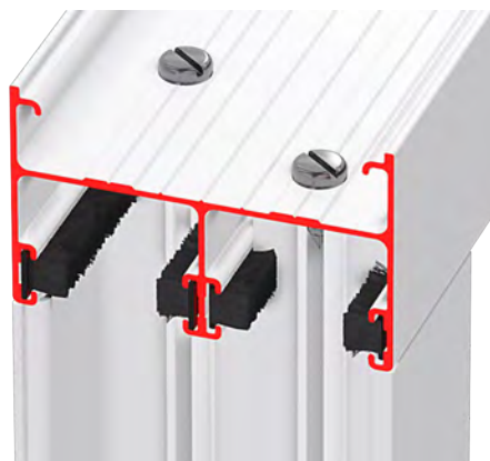
Armado Contramarco Horizontal Superior sin Venas
