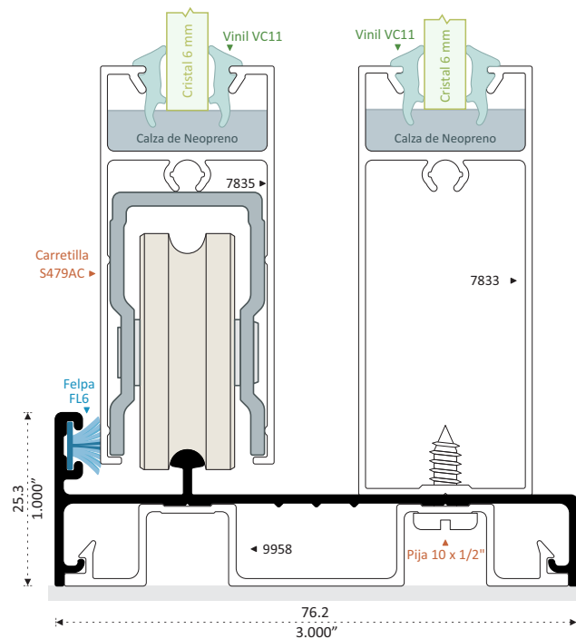
9957 RIEL Longitud 6.10 m
