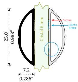
8272 MARQUETERÍA EXPUESTA CURVA Longitud 6.10 m
