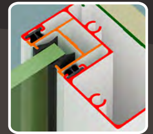
Cerco Fijo da Apariencia de un Perfil Integrado al Contramarco
