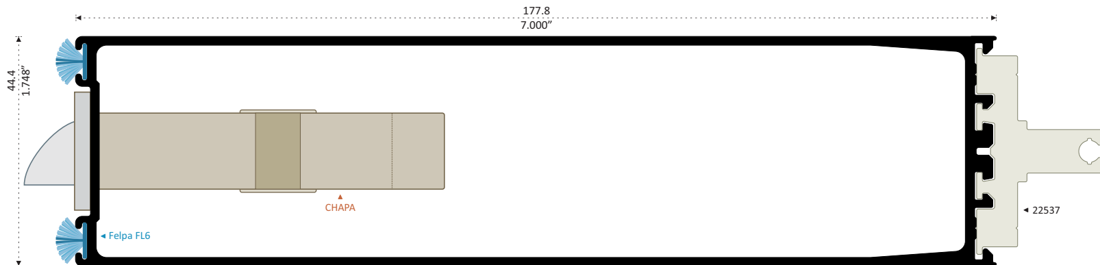
46901 PATENTE CERCO CHAPA Longitud: 5.00 m
