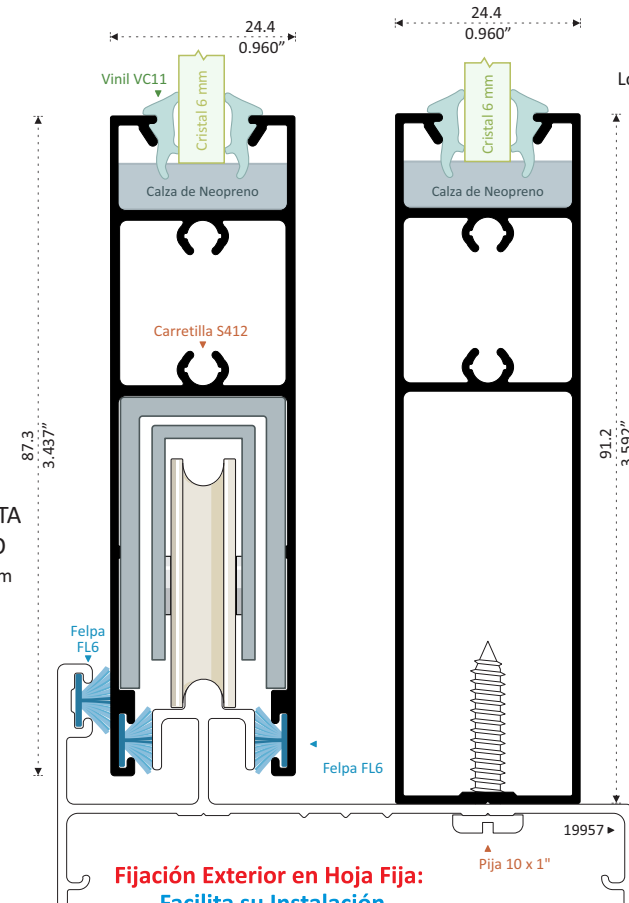
El Zoclo Entra hasta el Fondo del Traslape y Cerco Chapa Logrando Buena Hermeticidad
